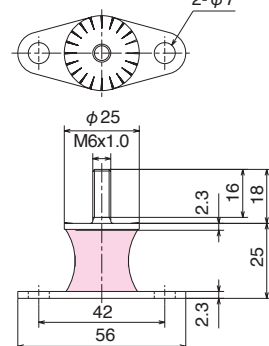
KXB-25-25H
