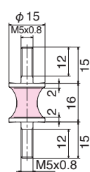
KXA-15-16H
