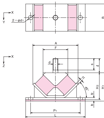
■ KC-75BP~100BP
