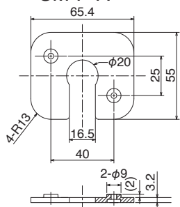
■ SM-20C~200C用 SM-P-A
