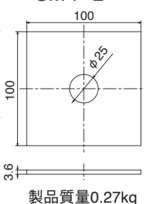
■ SM-300~450用 SM-P-L
