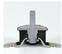
■ 断面写真
