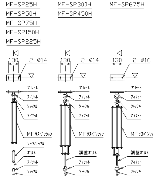
※MF リズバ'ンション (天吊りタイプ) 天井取付詳細
